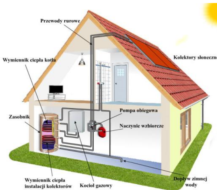
Ryc. 11. Schemat instalacji kolektorów słonecznych w domu jednorodzinnym
