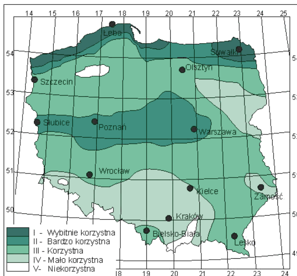
Ryc. 6. Strefy energetyczne wiatru w Polsce
