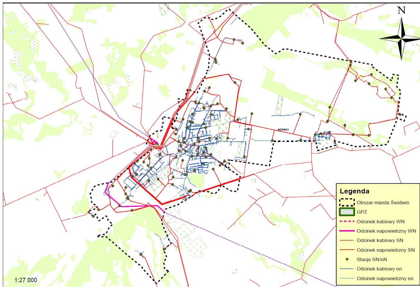
Ryc. 10. System elektroenergetyczny na obszarze miasta Świdwin
