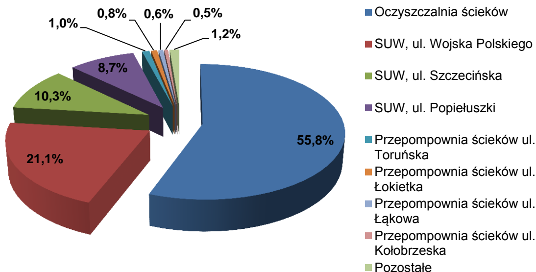
Wykres 29. Udział w zużyciu energii elektrycznej poszczególnych obiektów infrastruktury wodno-kanalizacyjnej
