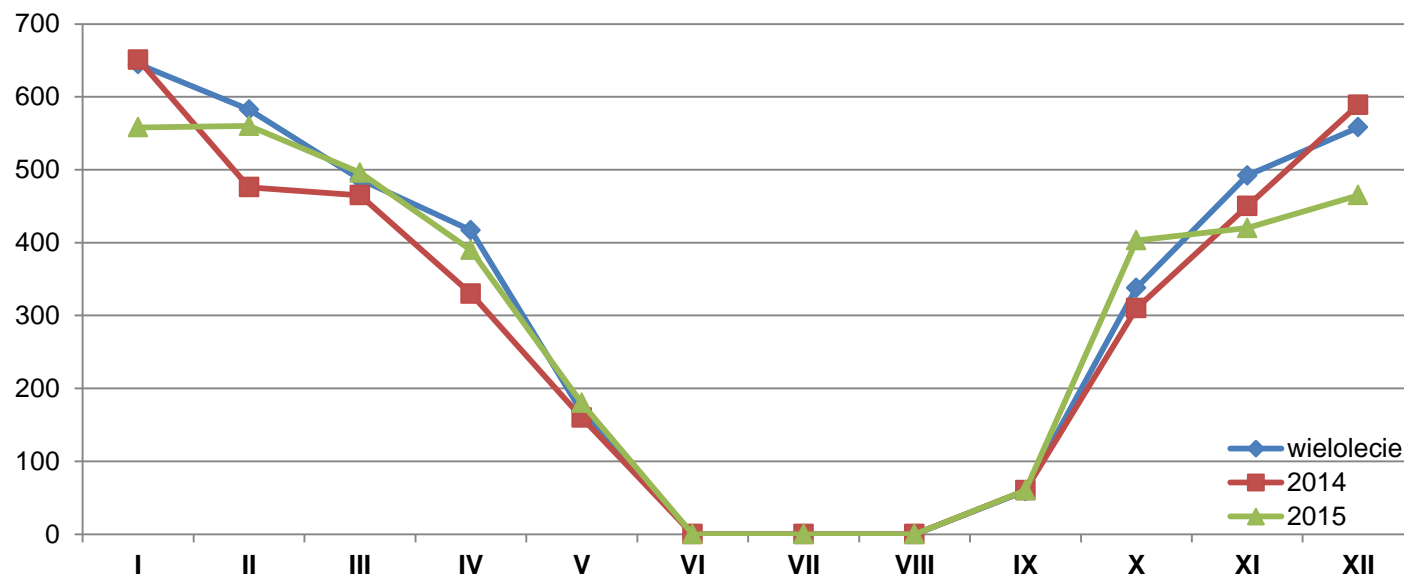
Wykres 3. Porównanie liczby stopniodni grzewczych w typowym roku meteorologicznym oraz w roku 2014 i 2015
