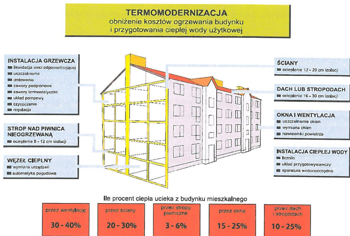
Ryc. 7. Termomodernizacja budynku
